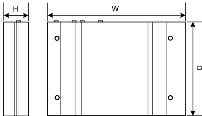
Fig. 1-2: Rappresentazione schematica, dimensioni in millimetri
